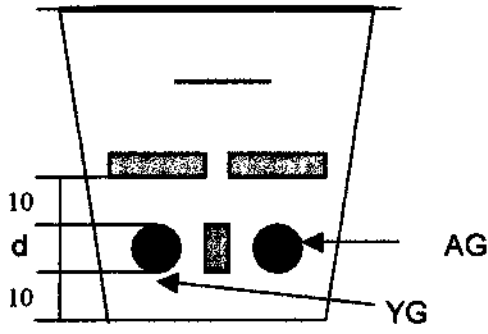
Şekil - 3 : AG ve YG(OG) kabloların Yanyana dşenmesi
