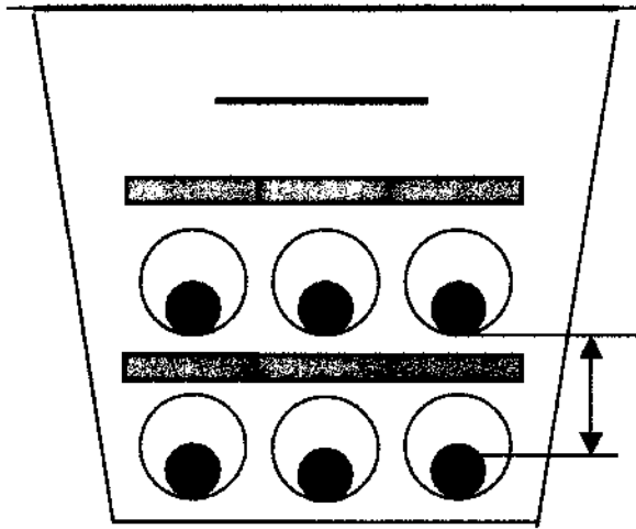
Şekil 4.a: Kabloların boru içinde montajı
