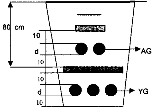
Şekil - 4 : AG ve YG(OG) kabloların Altı üstlü dşenmesi
