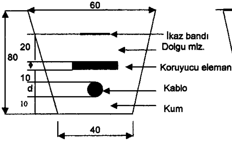
Şekil-1: Standart Kablo Kanalı
