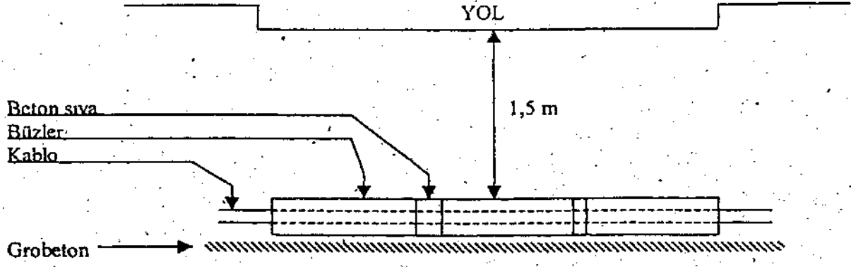
( Şekil - 7 ) Büzlü geçiş
