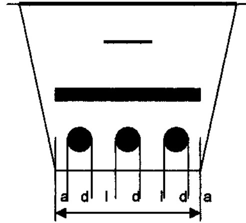
Şekil-2-a : Birden fazla AG veya YG(OG) Döşenmesi ve hesap örneği
